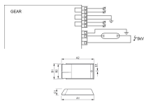
Scheda tecnica Philips HID-PV C 50 /I CDM 220-240V 50/60Hz
